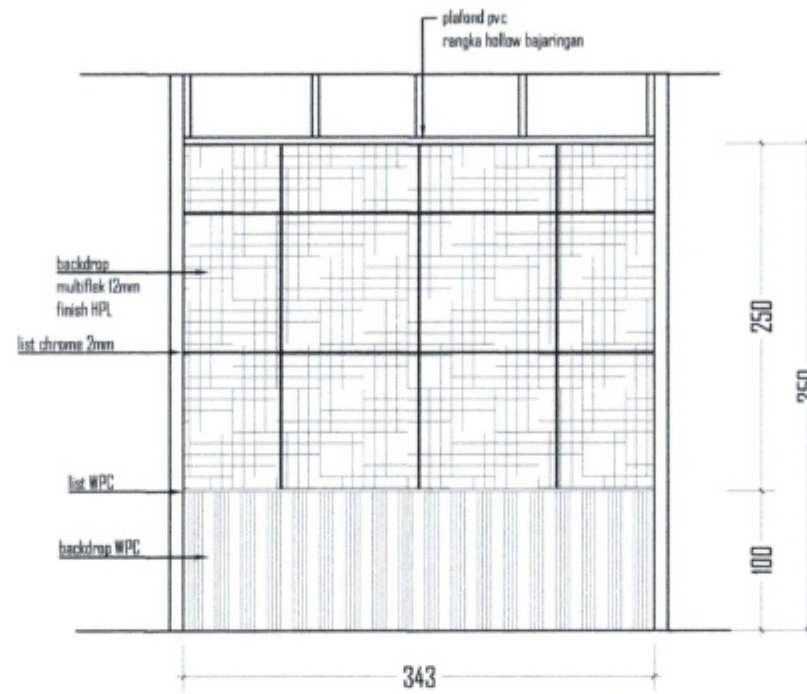
POTONGAN BANGUNAN
