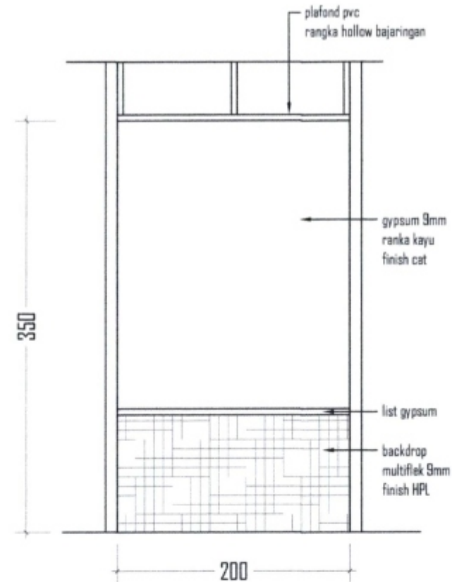
POTONGAN BANGUNAN
