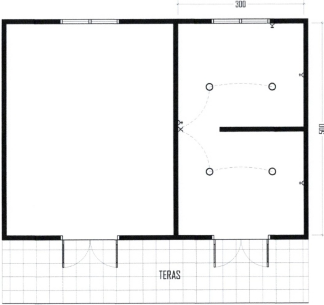
DENAH ELEKTRIKAL
