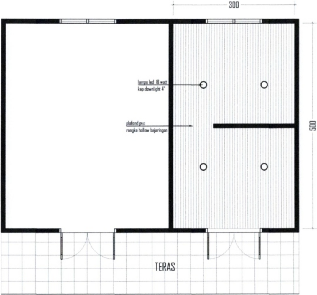
DENAH PLAFOND
