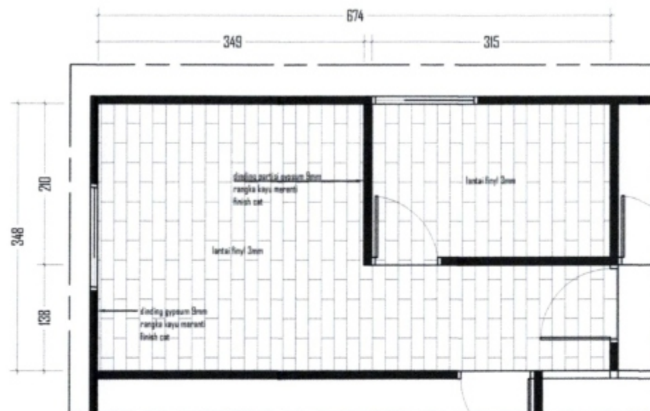
DENAH RENCANA RUANG BERMAIN ANAK DAN RUANG PENGADUAN MASYARAKAT
