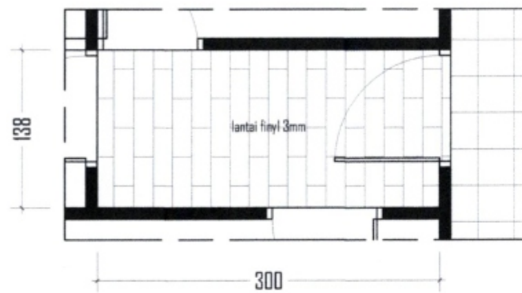
DENAH RENCANA RUANG LOBBY KANTOR
