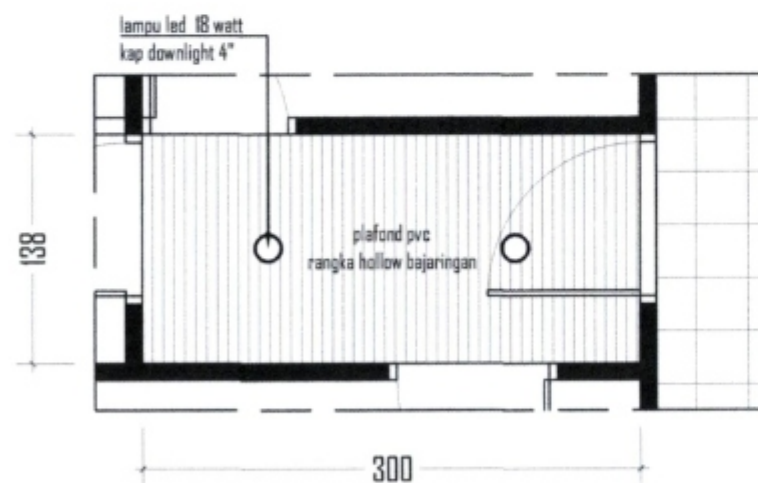
DENAH RENCANA PLAFOND
