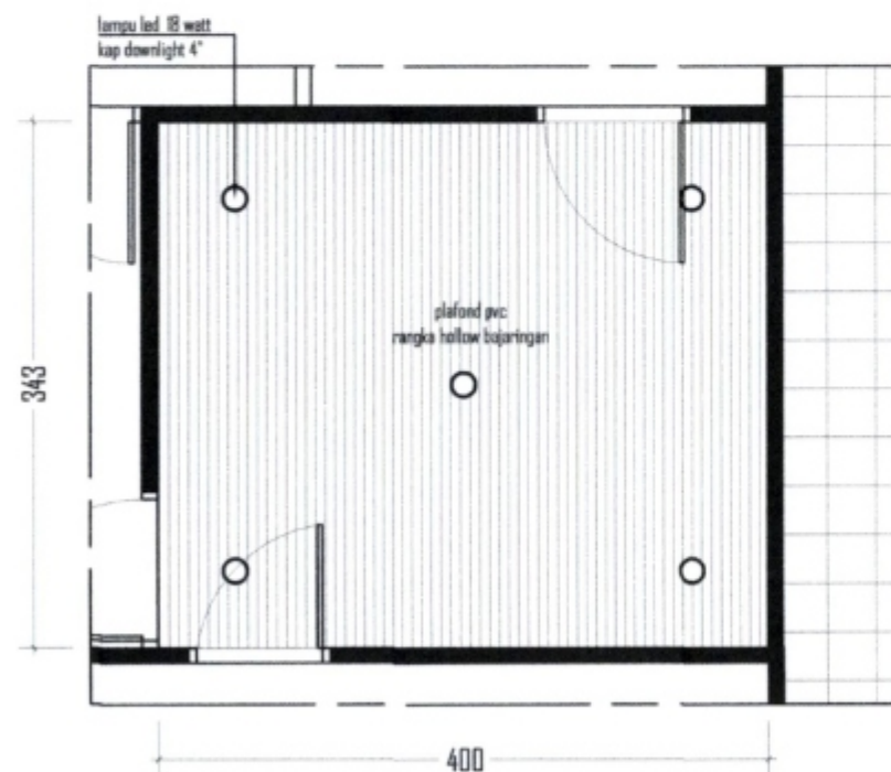
DENAH RENCANA PLAFOND
