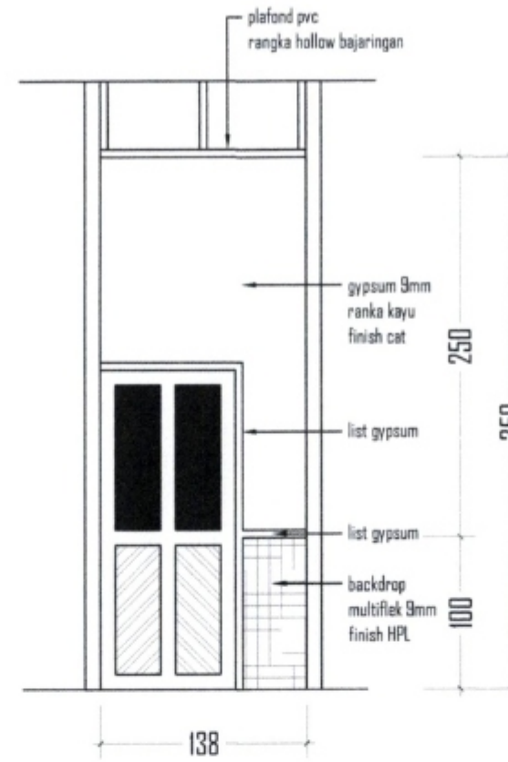
POTONGAN BANGUNAN
