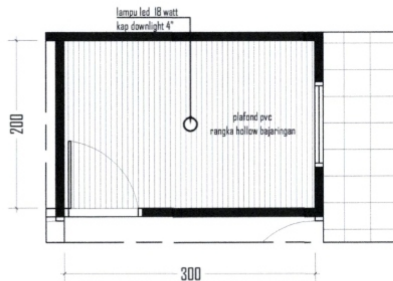
DENAH RENCANA PLAFOND
