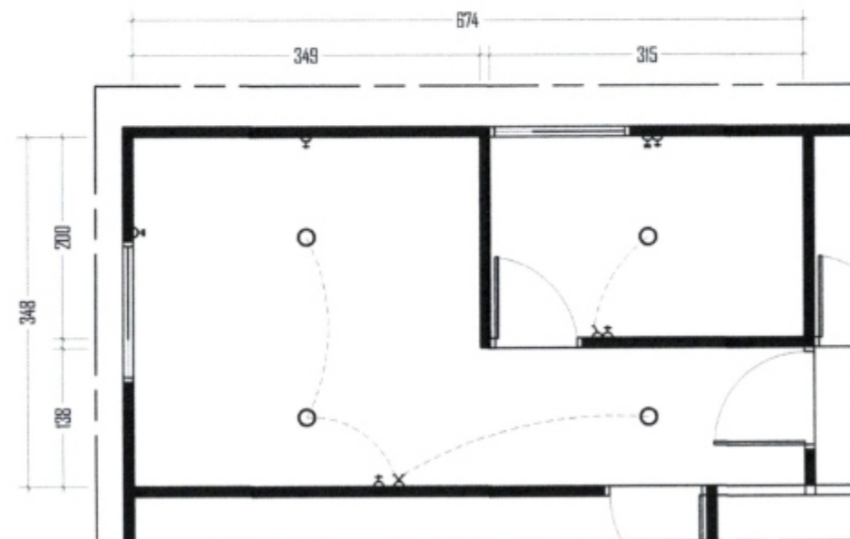
DENAH RENCANA ELEKTRIKAL
