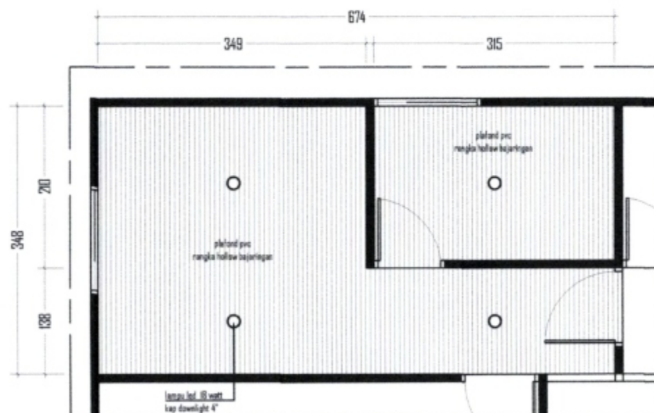
DENAH RENCANA PLAFOND
