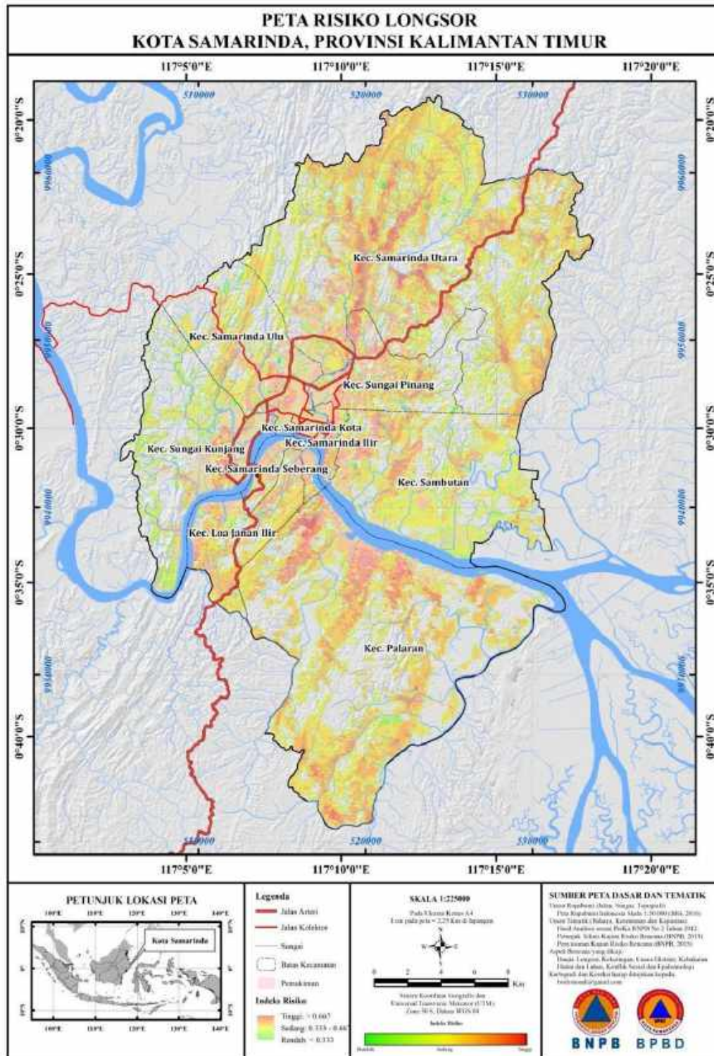
Gambar 2.33. Peta Risiko Longsor Kota Samarinda
