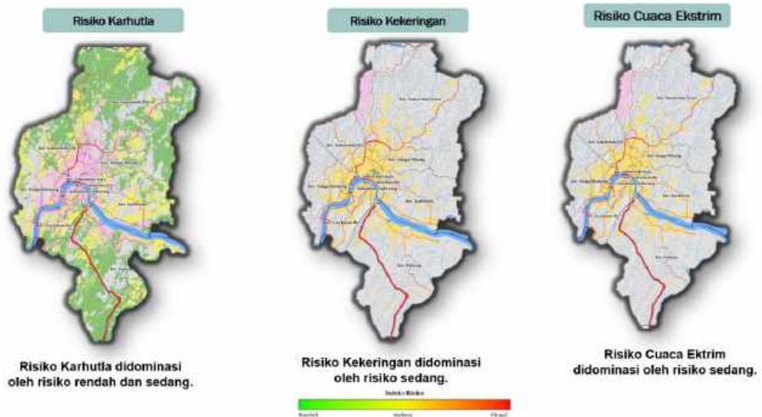
Gambar 2.34. Risiko karhutla, kekeringan dan cuaca ekstrim
