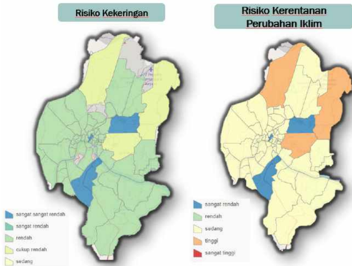
Gambar 2.40. Indeks kerentanan terhadap perubahan iklim Kota Samarinda
