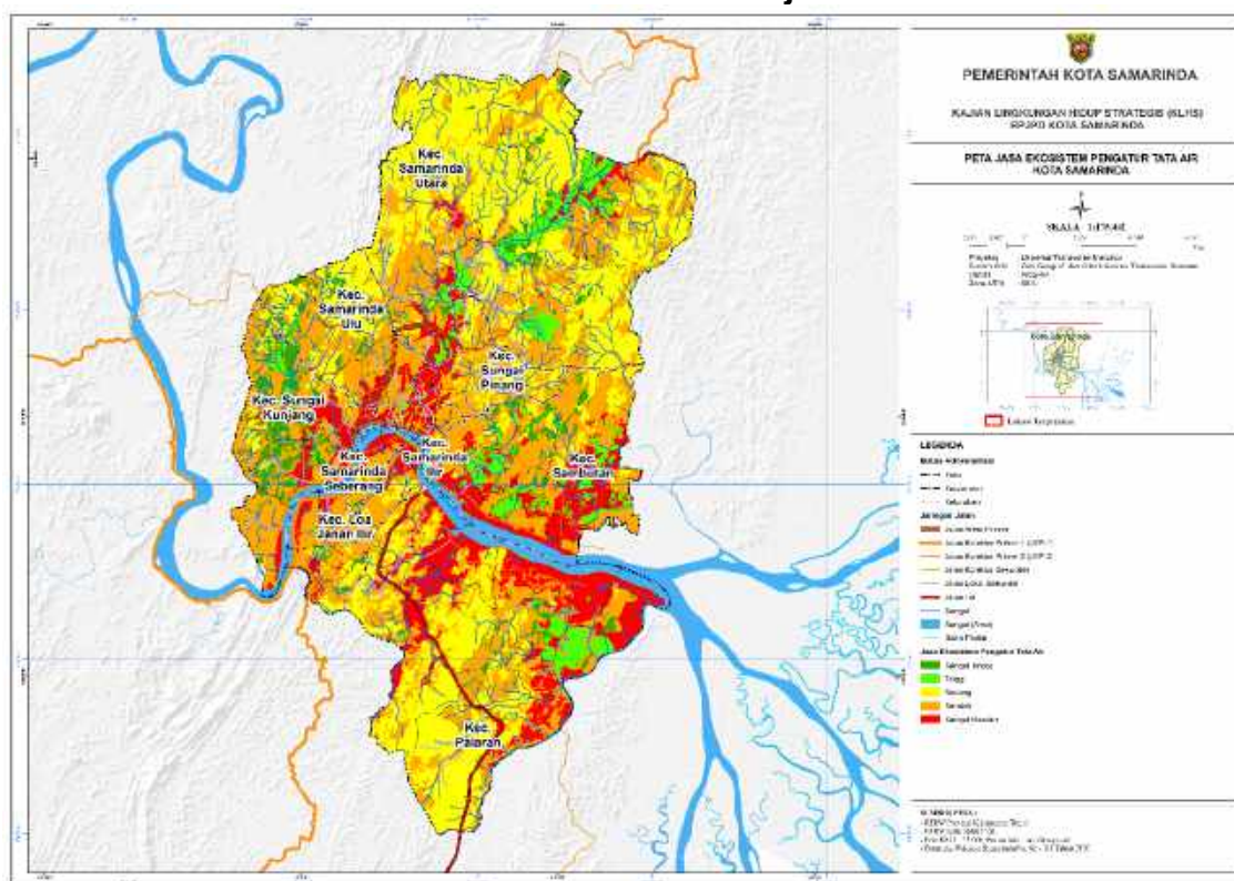
Gambar 2.37. Jasa ekosistem tata aliran air dan banjir Kota Samarinda
