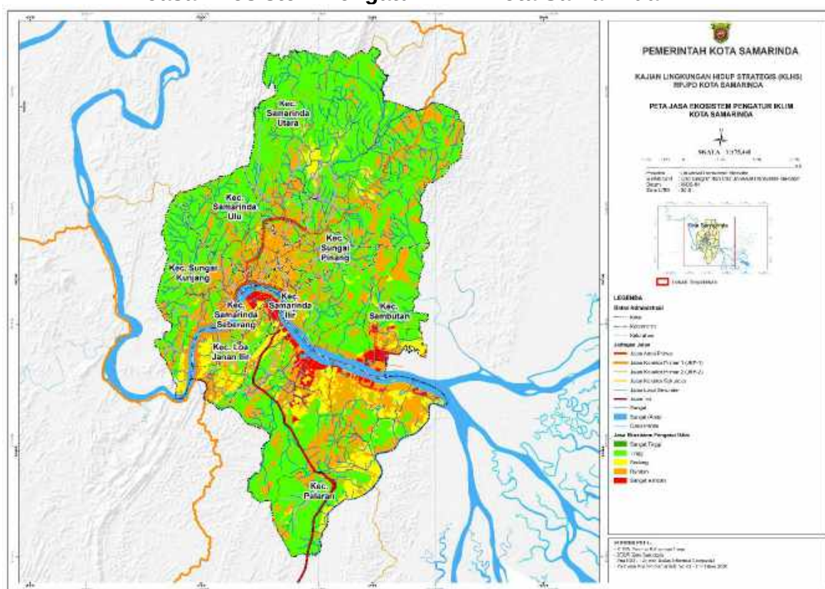
Gambar 2.38. Jasa Ekosistem Pengatur Iklim Kota Samarinda
