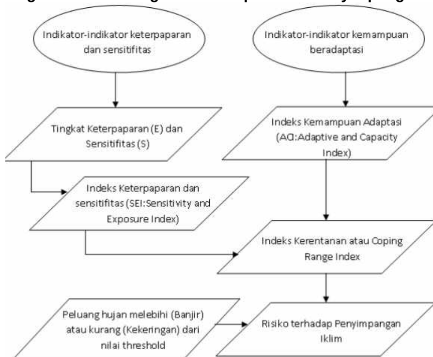
Gambar 2.39. Kerangka Berfikir Kategori Terhadap Resiko Penyimpangan Iklim
