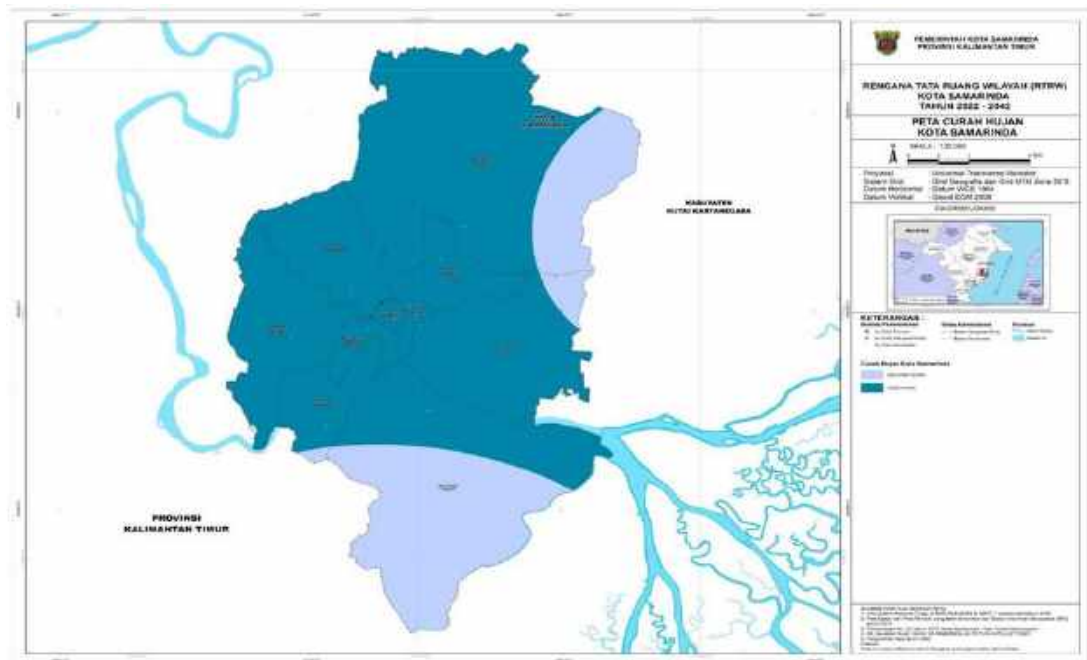
Gambar 2.5. Peta Curah Hujan Kota Samarinda
